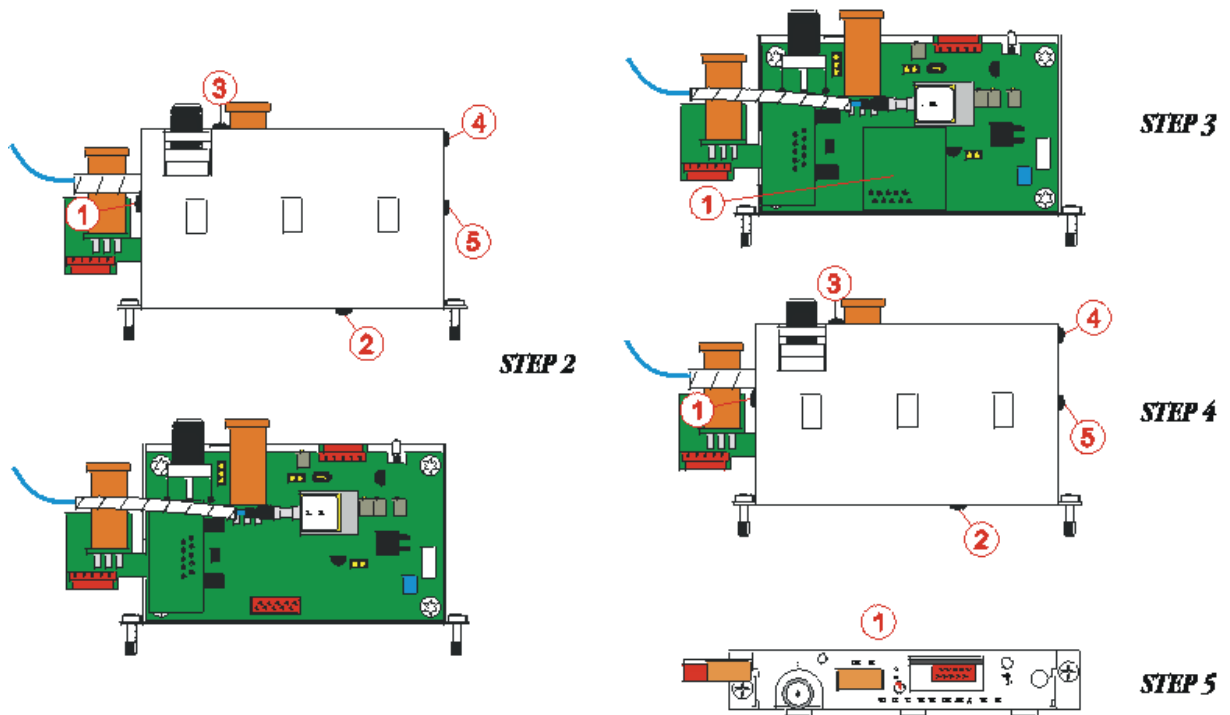
Fig. 17. RRG xxx module installation.
