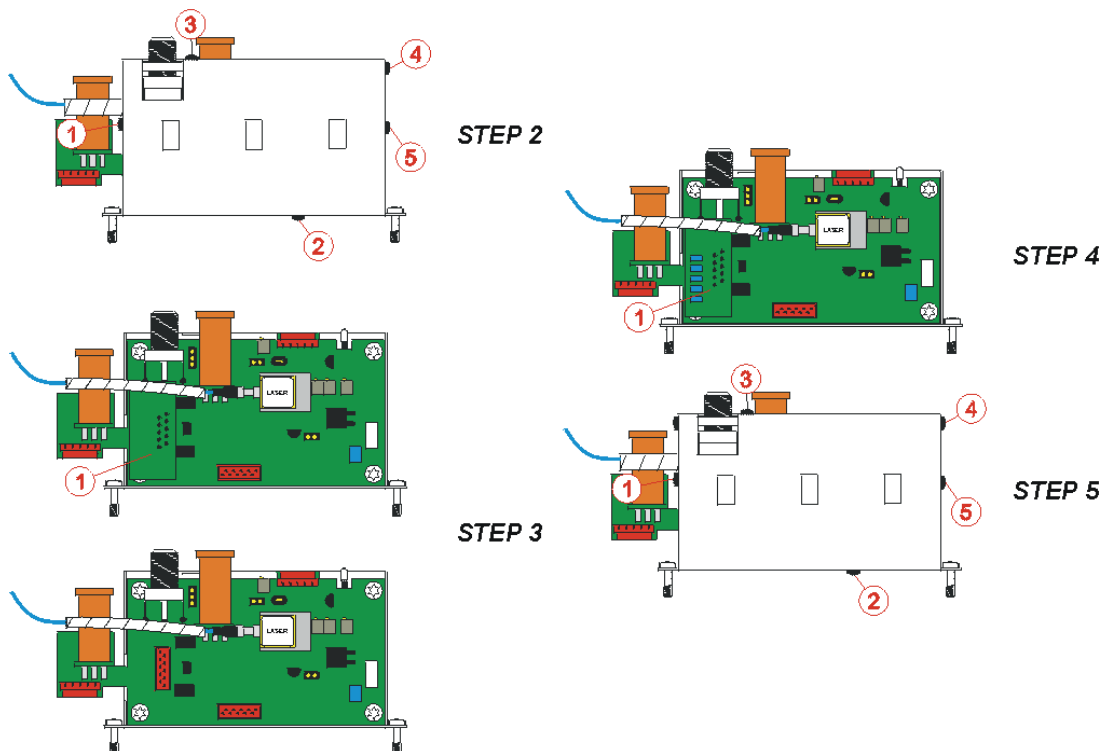
Fig. 16. OLPA xx module installation.
